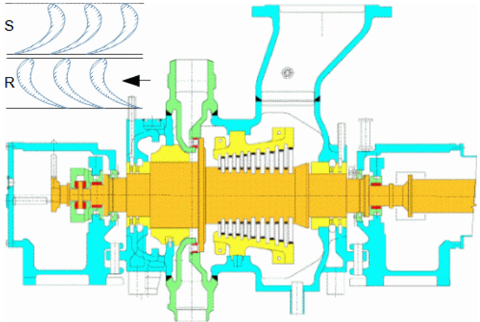
170: 6 MW 10-stupňová parní turbína
